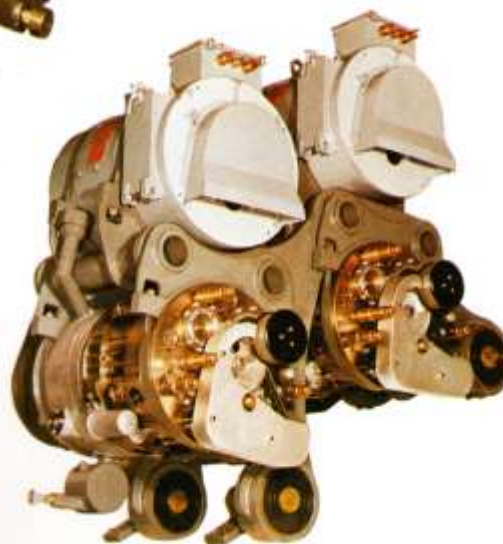
COMPRESSEUR HAUTE PRESSION DE SOUS-MARIN TGM 60/100
